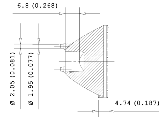
Sez. A-A
