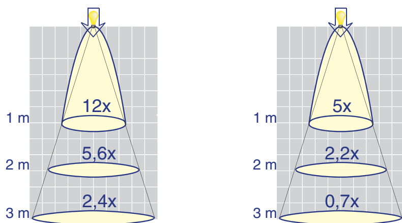
KEPL2425 (25°)
